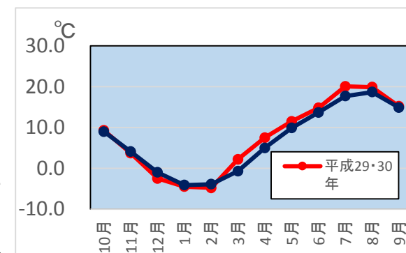
図-1 平成 29 年 10 月～30 年 9 月平均気温（奥日光）
