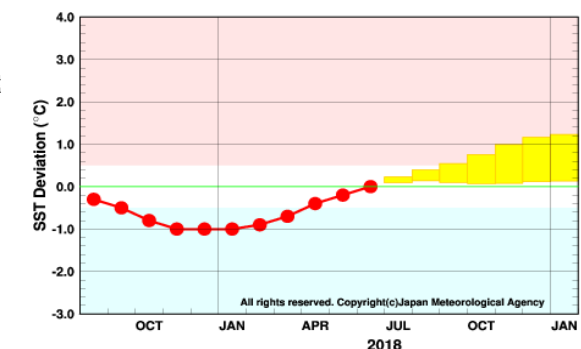
図-2 エルニーニョ／ラニーニャ現象の経過と予測（気象庁）
