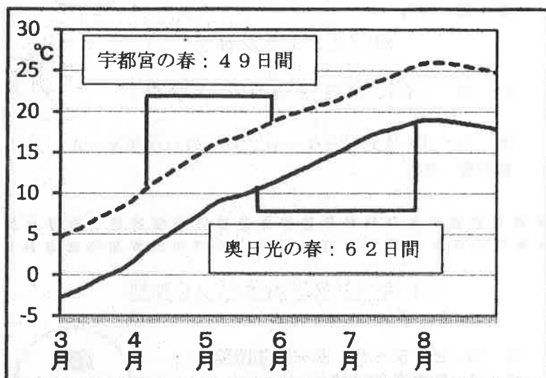
春～夏の気温の推移 (点線：宇都宮、実線：奥日光)
